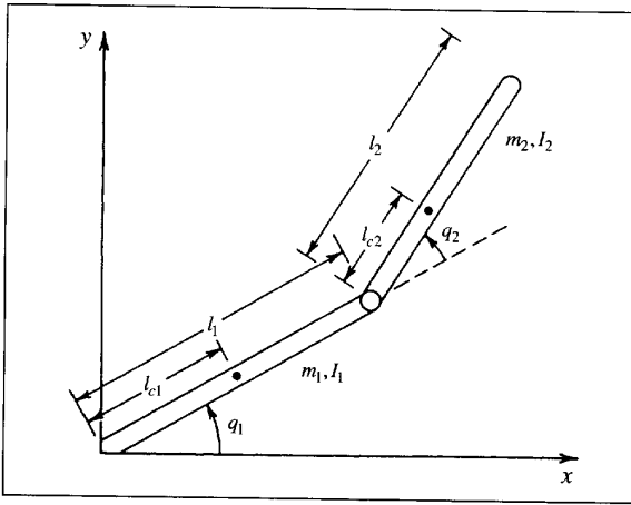
Fig. 1. The Acrobot.
